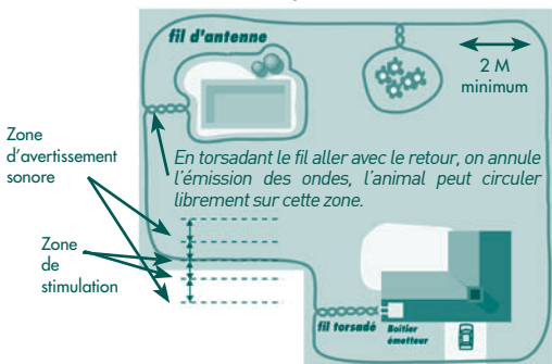
Schéma 4 exemple d'installation
