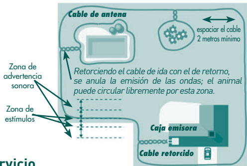
Esquema nº 4: Ejemplo de instalación
